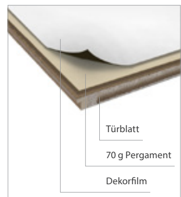
Detail Oberflächenaufbau
