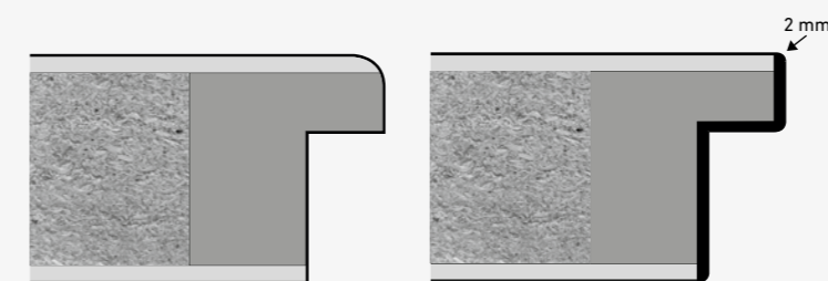
STANDARDKANTE (RP) CHANT STANDARD (RP)
